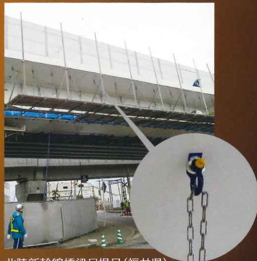
北陸新幹線橋梁足場吊(福井県)
