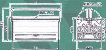
■ BX230 ケース寸法
